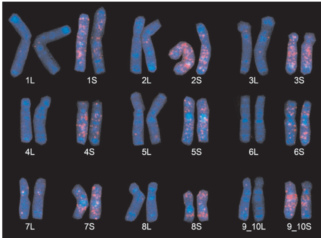
図5. アフリカツメガエルのサブゲノムの同定。サブゲノム S に特異的な“化石化” DNA 配列を用いて、染色体（青）を FISH 法で赤く染色したもの。染色体 1 番～9 番（9_10 番）の S の染色体により多くの赤い染色が見られる。これらは祖先種 S に由来したものと考えられる。9 番目の染色体は、ネッタイツメガエルの 9 番と 10 番染色体が融合した染色体に相当するため染色体 9_10 番と呼ぶ。
