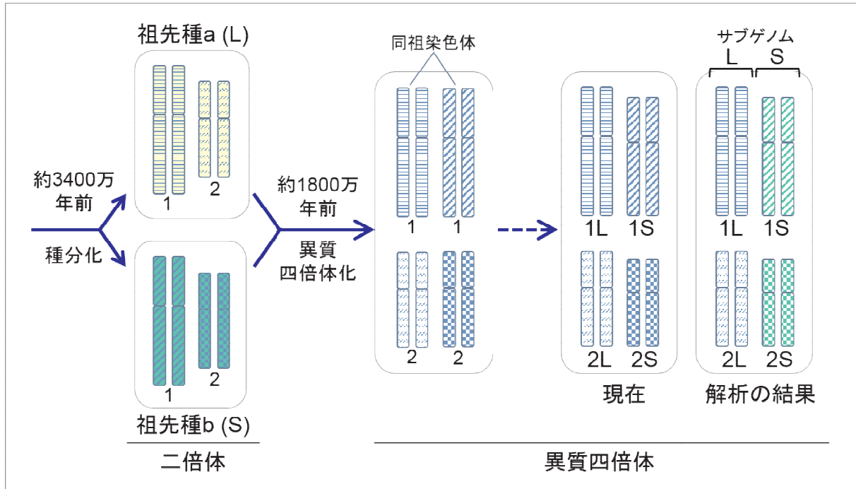
図4. 異質四倍体は祖先種に由来する2つのサブゲノムをもつ。ここでは簡単にするため祖先種aとbの染色体は1番と2番の2対のみを描いた（実際は祖先種は9対でアフリカツメガエルは18対である）。異質四倍体化の直後は、同祖染色体間に区別がないが現在までに一方が短くなったと考えられる。そこで長い方をL (long)、短い方をS (short)と命名した。今回、詳細なゲノム解析を行った結果、染色体LのセットとSのセットが、祖先種由来のゲノム（これをサブゲノムという）にそれぞれ対応することが示された。そこで、二つのサブゲノムをLとSと命名し、さらに祖先種もLとSと命名した。この発見により、倍数化後のサブゲノムの変化を解析することが可能となった。
